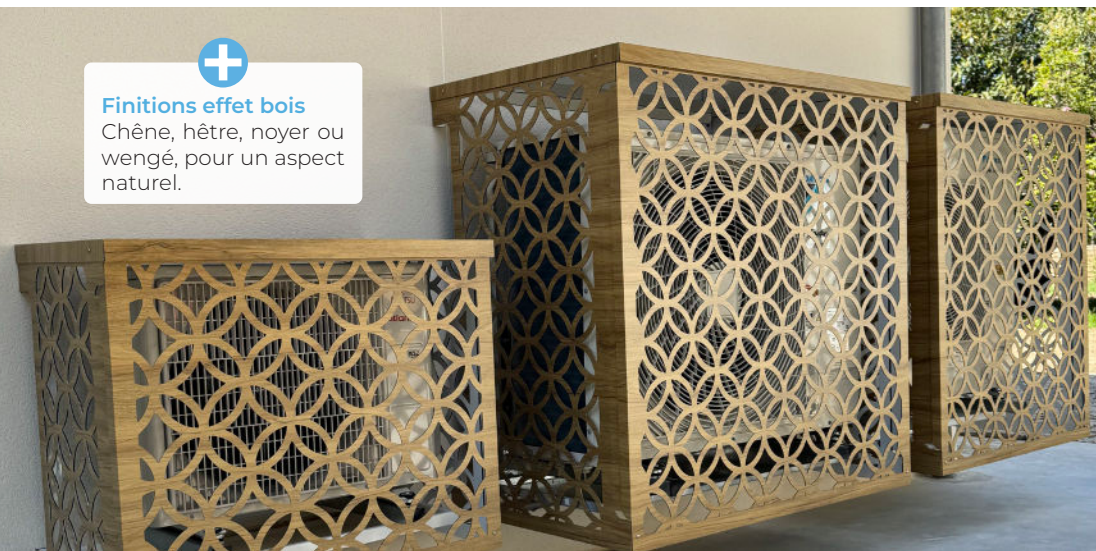
Échancrures latérales et supérieures pour la ventilation et le passage des goulottes
